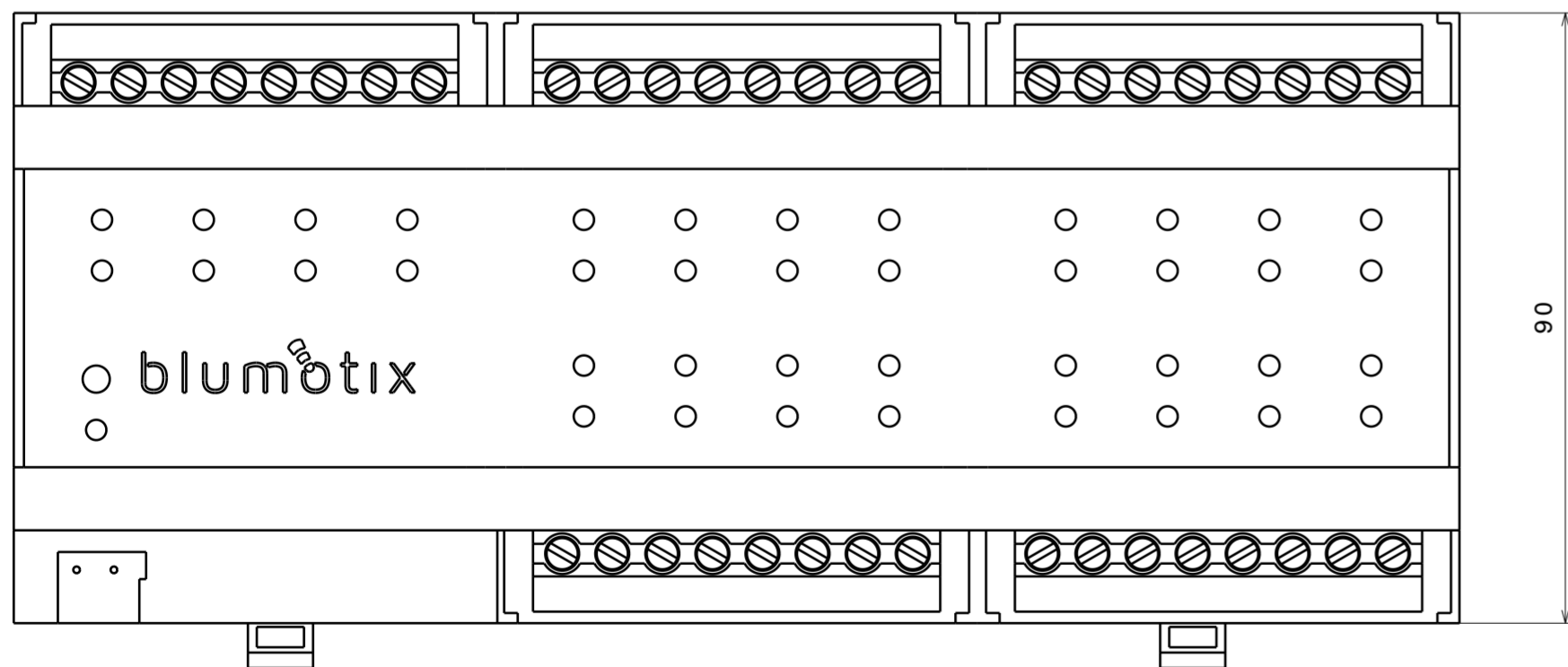
Vista dall'alto Scala: 1:1
