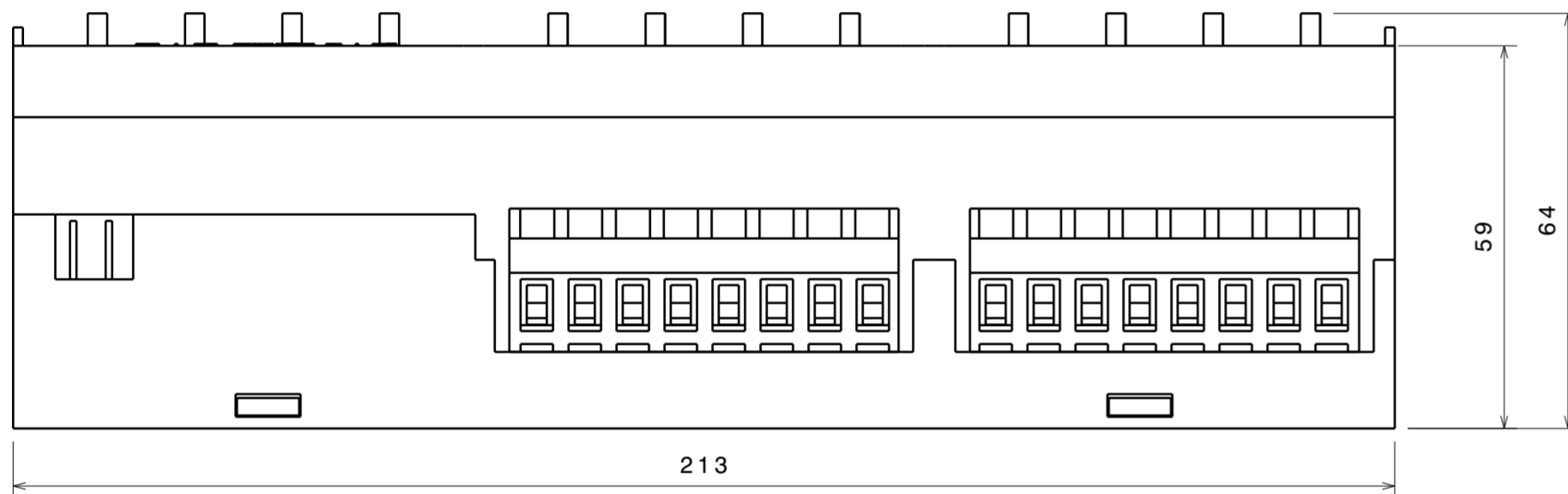
Vista frontale Scala: 1:1
