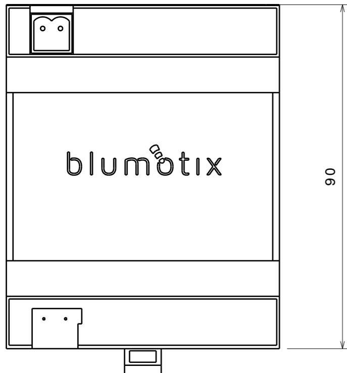
Vista dall'alto Scala: 1:1
