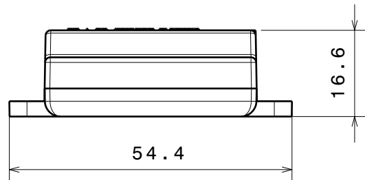
Vista frontale Scala: 1:1
