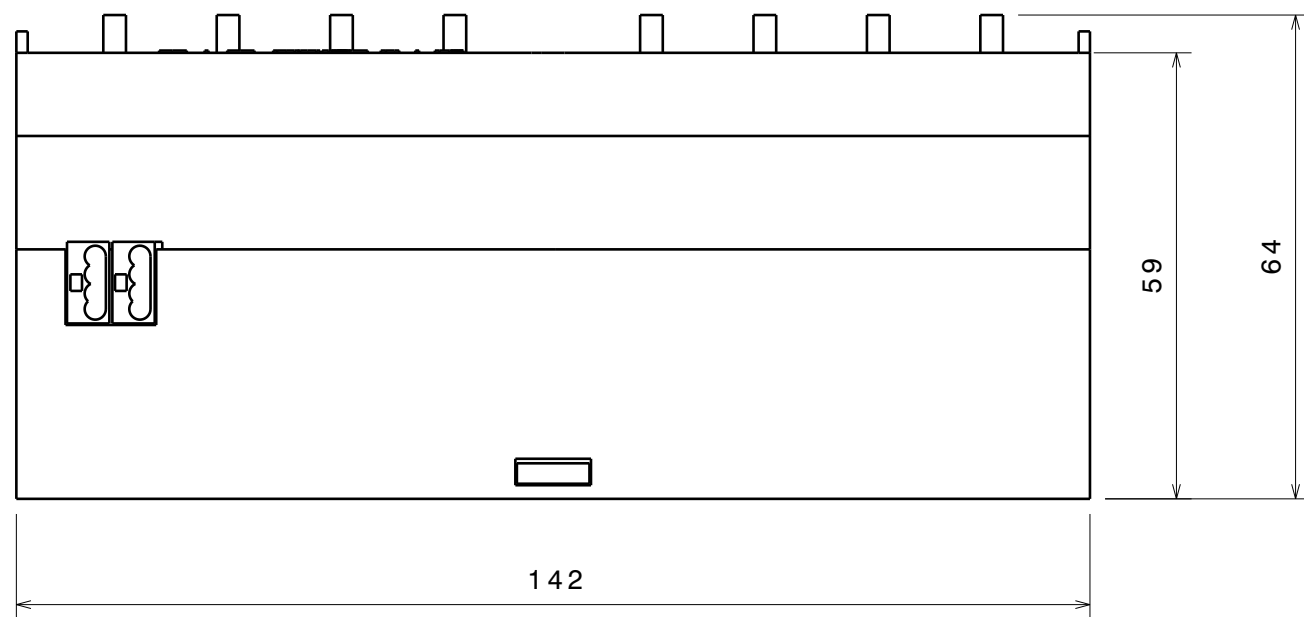
Vista frontale Scala: 1:1
