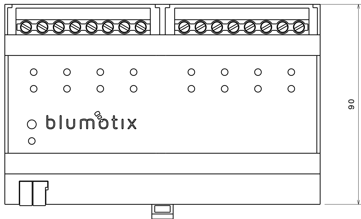
Vista dall'alto Scala: 1:1
